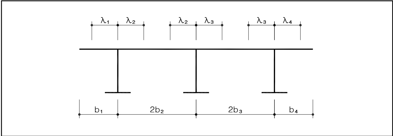
【그림 6.2.3】 플랜지의 유효폭(대구)
