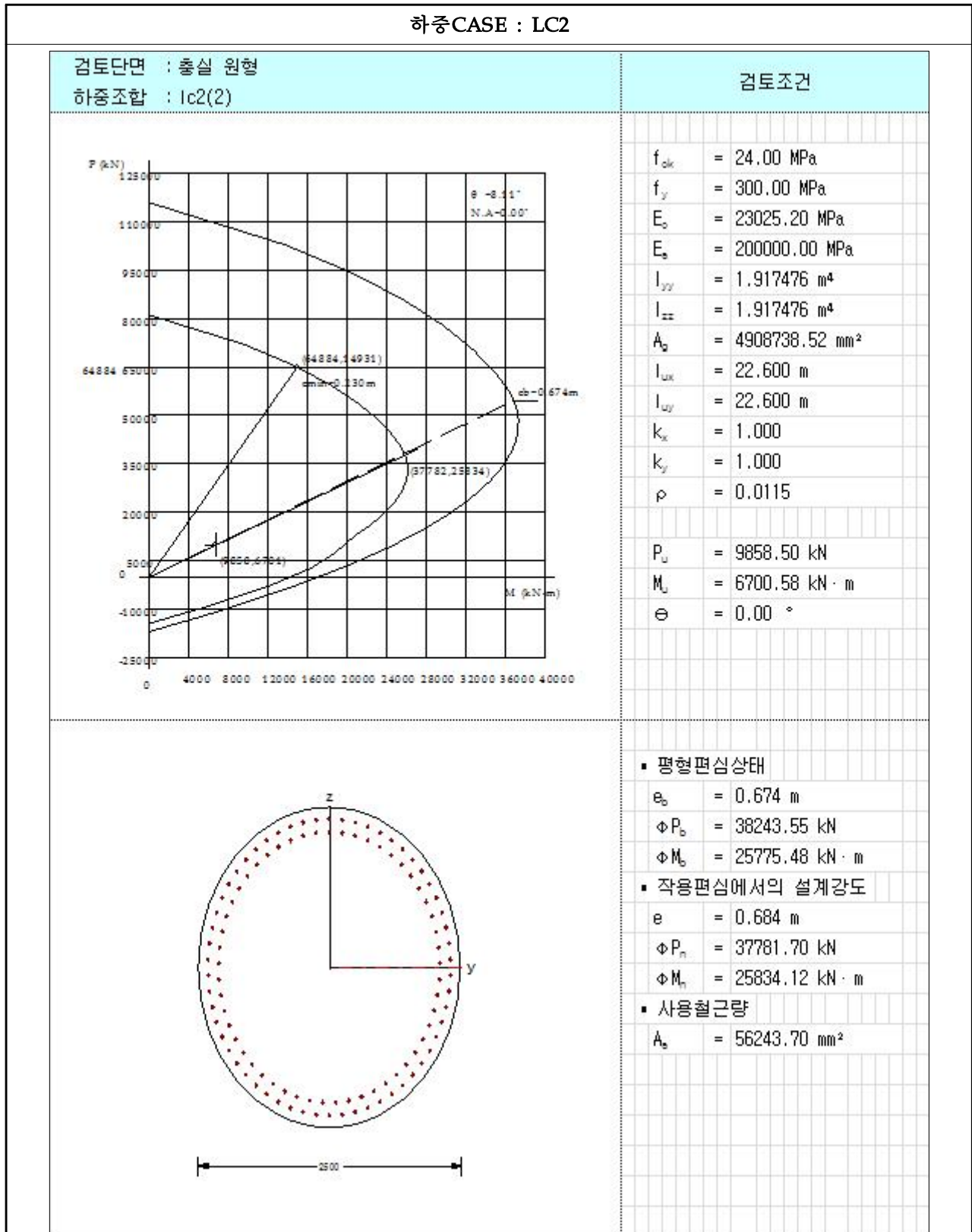
【그림 6.4.4】 P-M 상관도(하중CASE : LC2)(대구)
