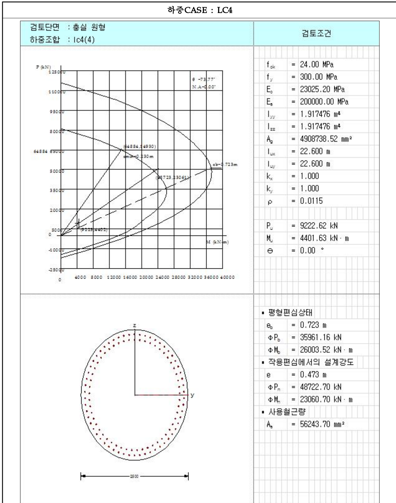
【그림 6.4.26】 P-M 상관도(하중CASE : LC4)(부산)
