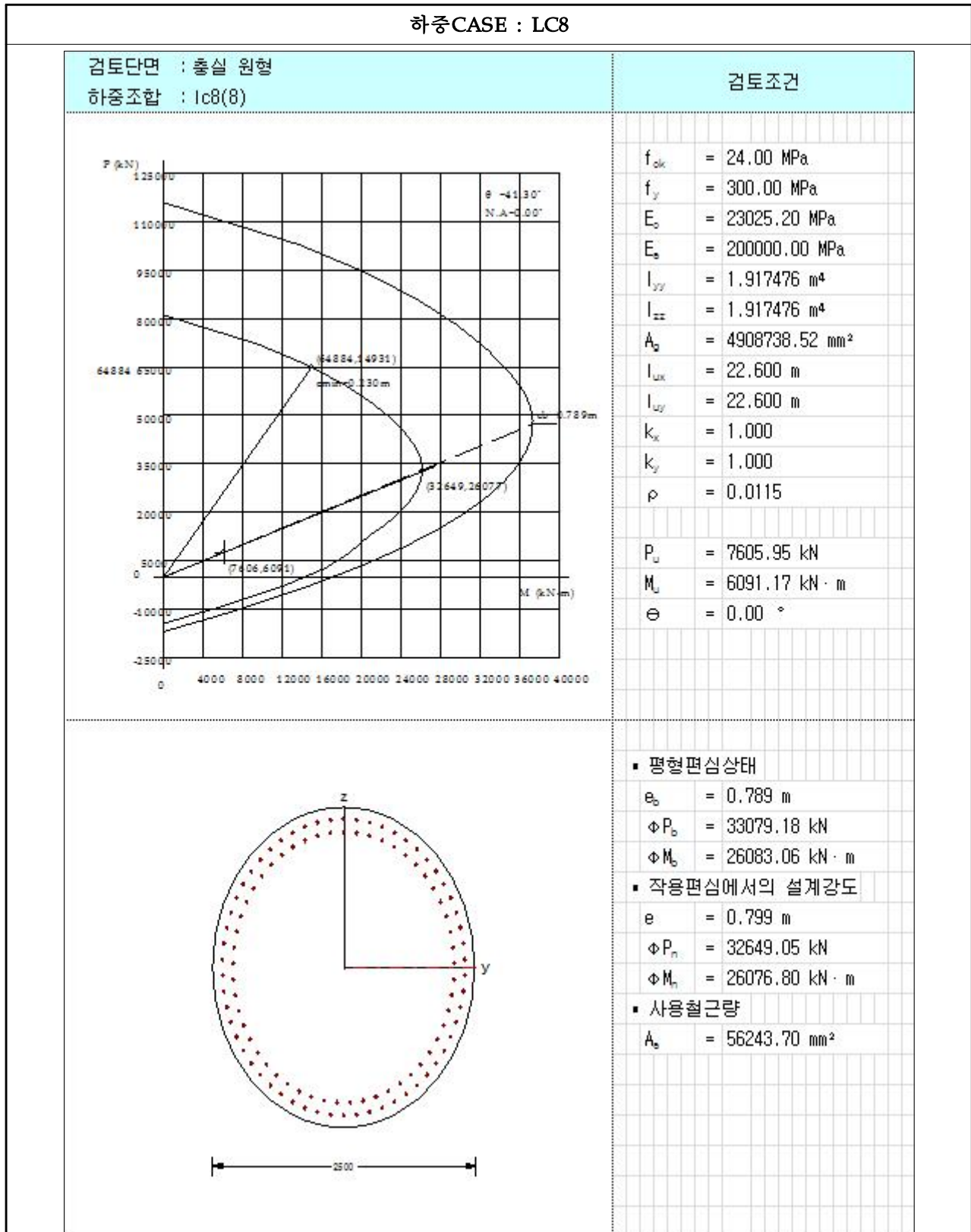
【그림 6.4.39】 P-M 상관도(하중CASE : LC8)(부산)
