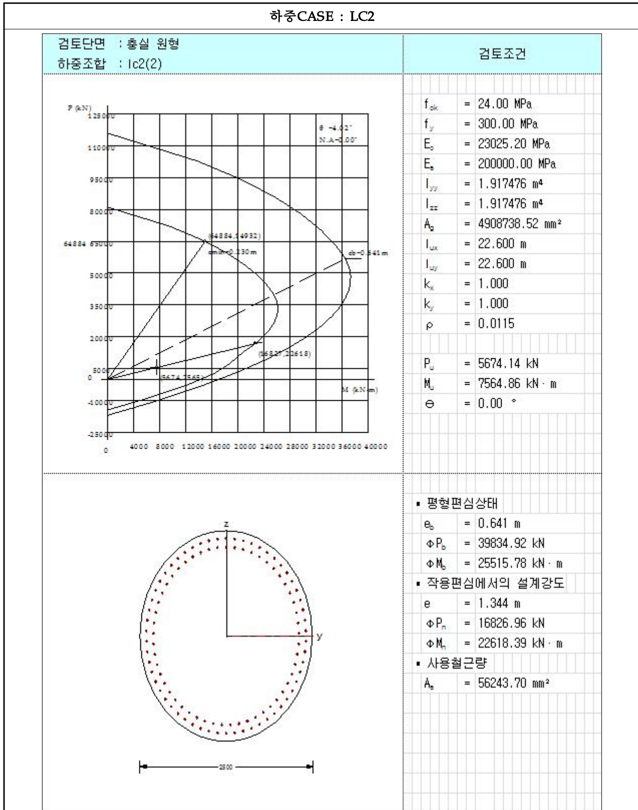
【그림 6.4.13】 P-M 상관도(하중CASE : LC2)(대구)
