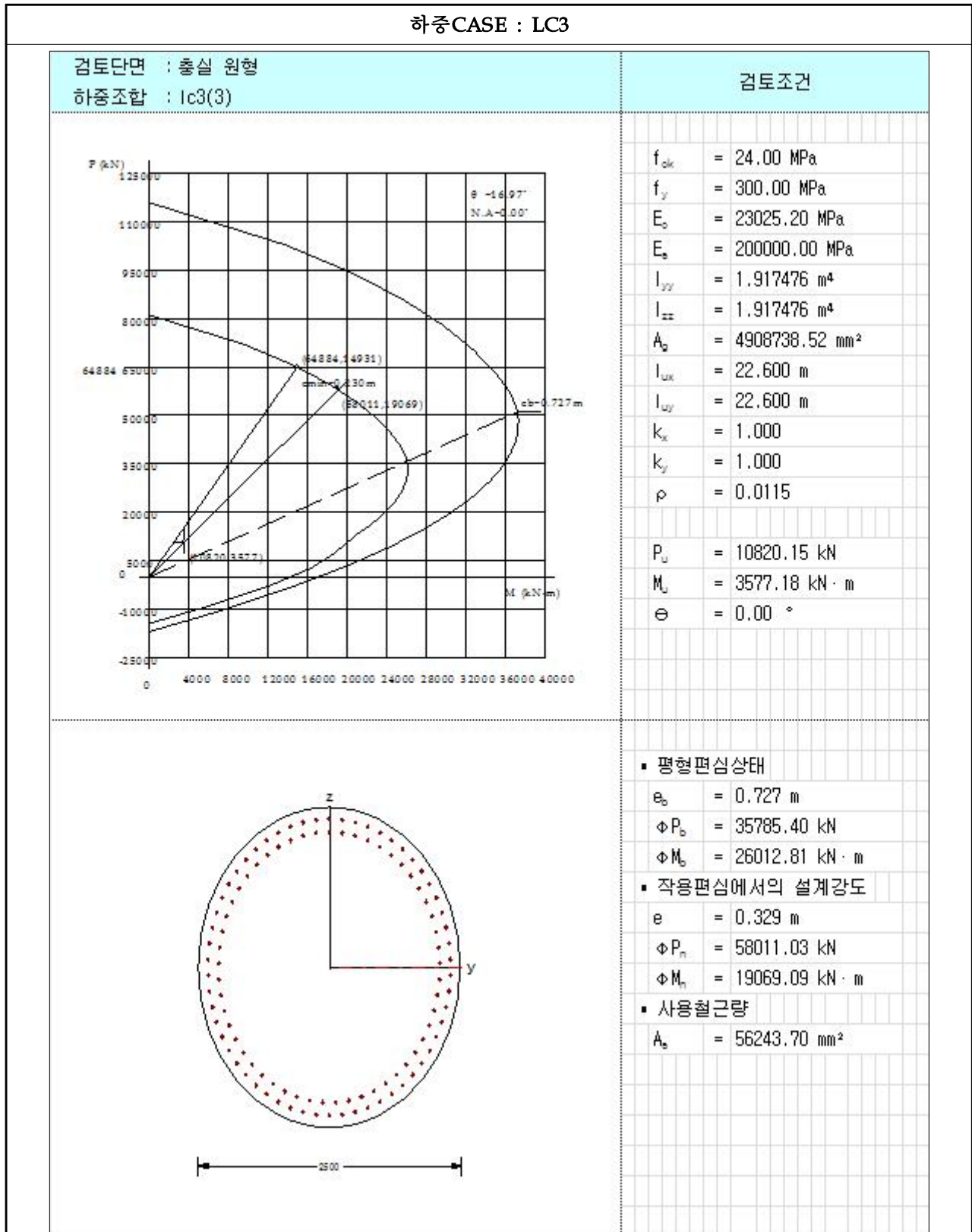
【그림 6.4.5】 P-M 상관도(하중CASE : LC3)(대구)
