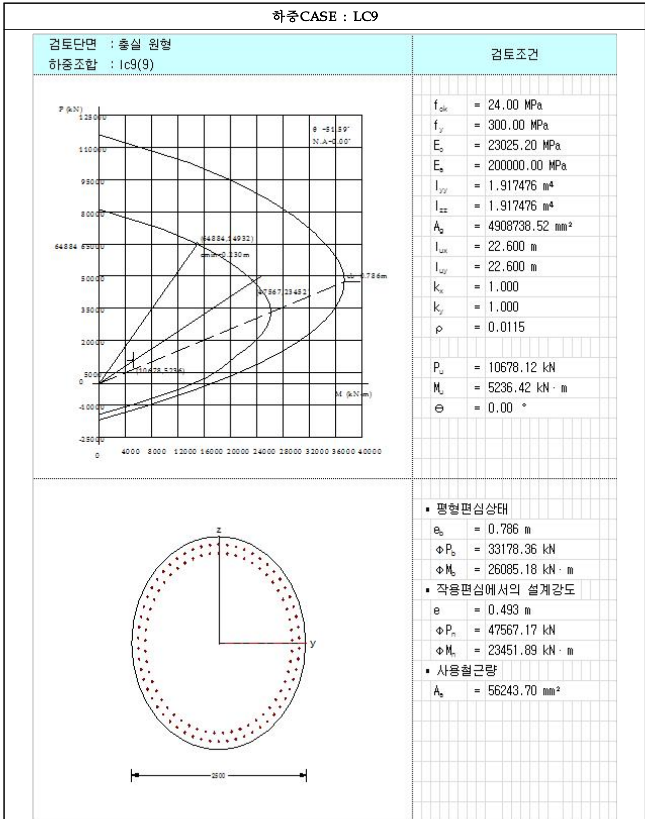
【그림 6.4.11】 P-M 상관도(하중CASE : LC9)(대구)
