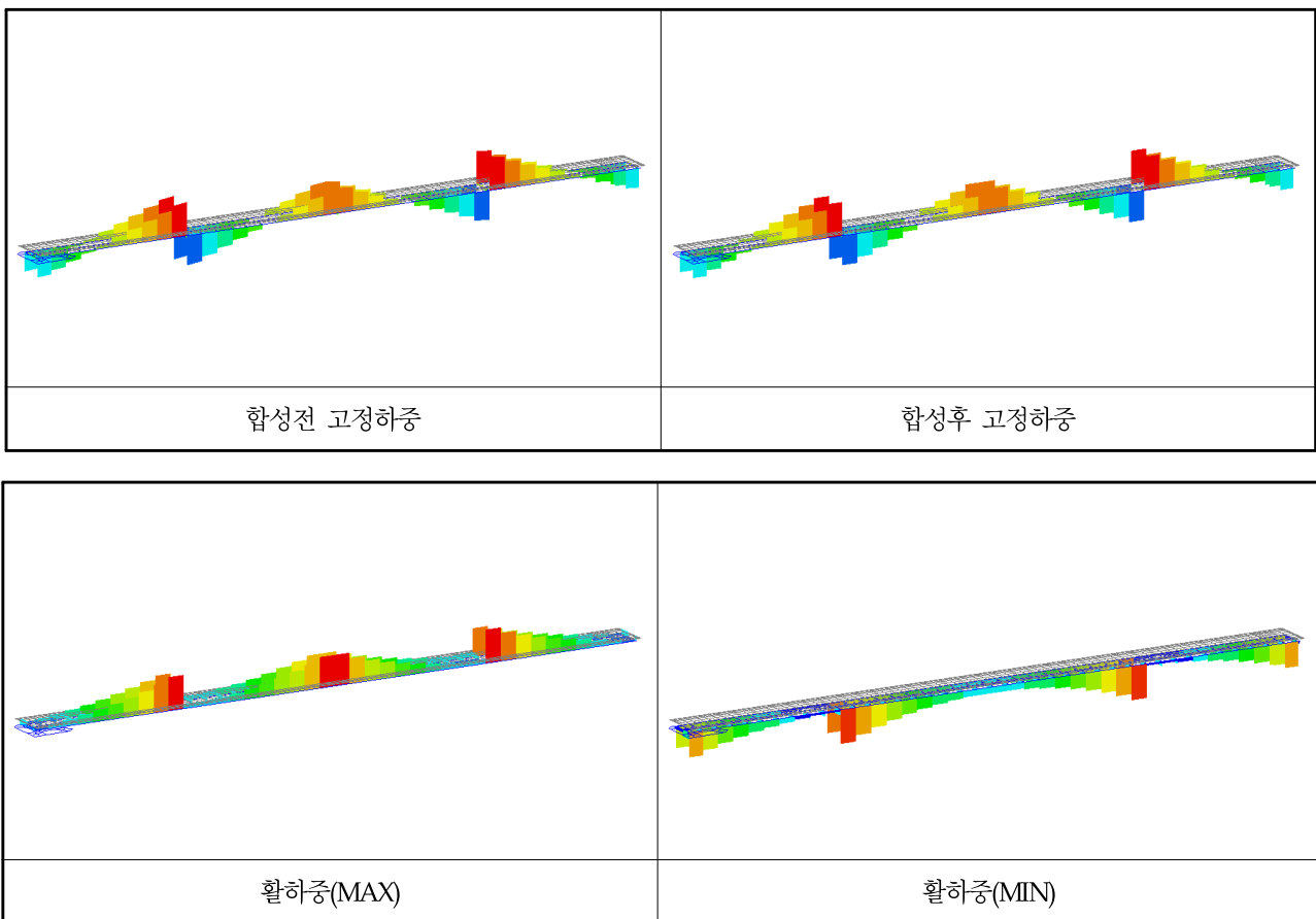
【그림 6.2.20】 전단력도(부산)
