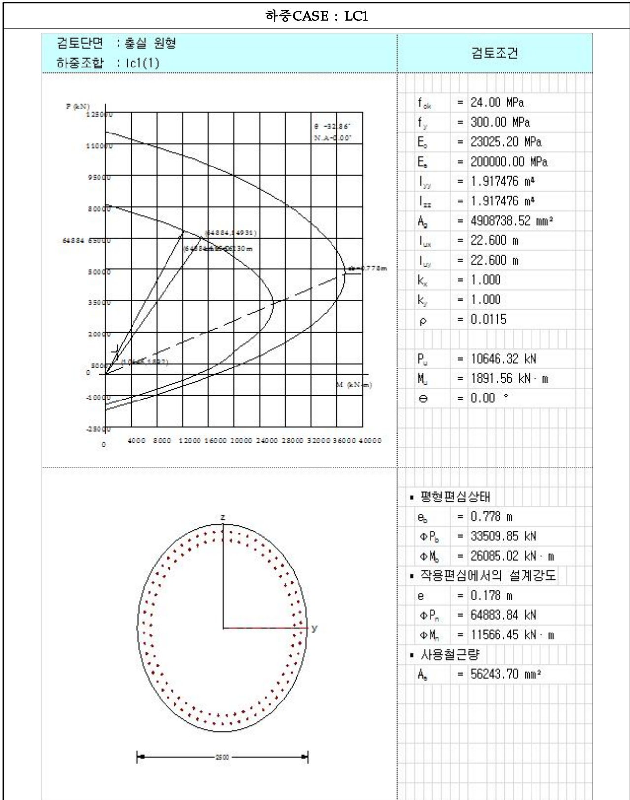
【그림 6.4.12】 P-M 상관도(하중CASE : LC1)(대구)
