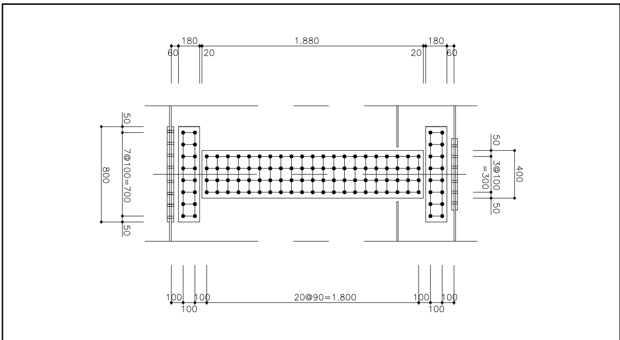
【그림 6.2.23】 Web 이음(부산)
