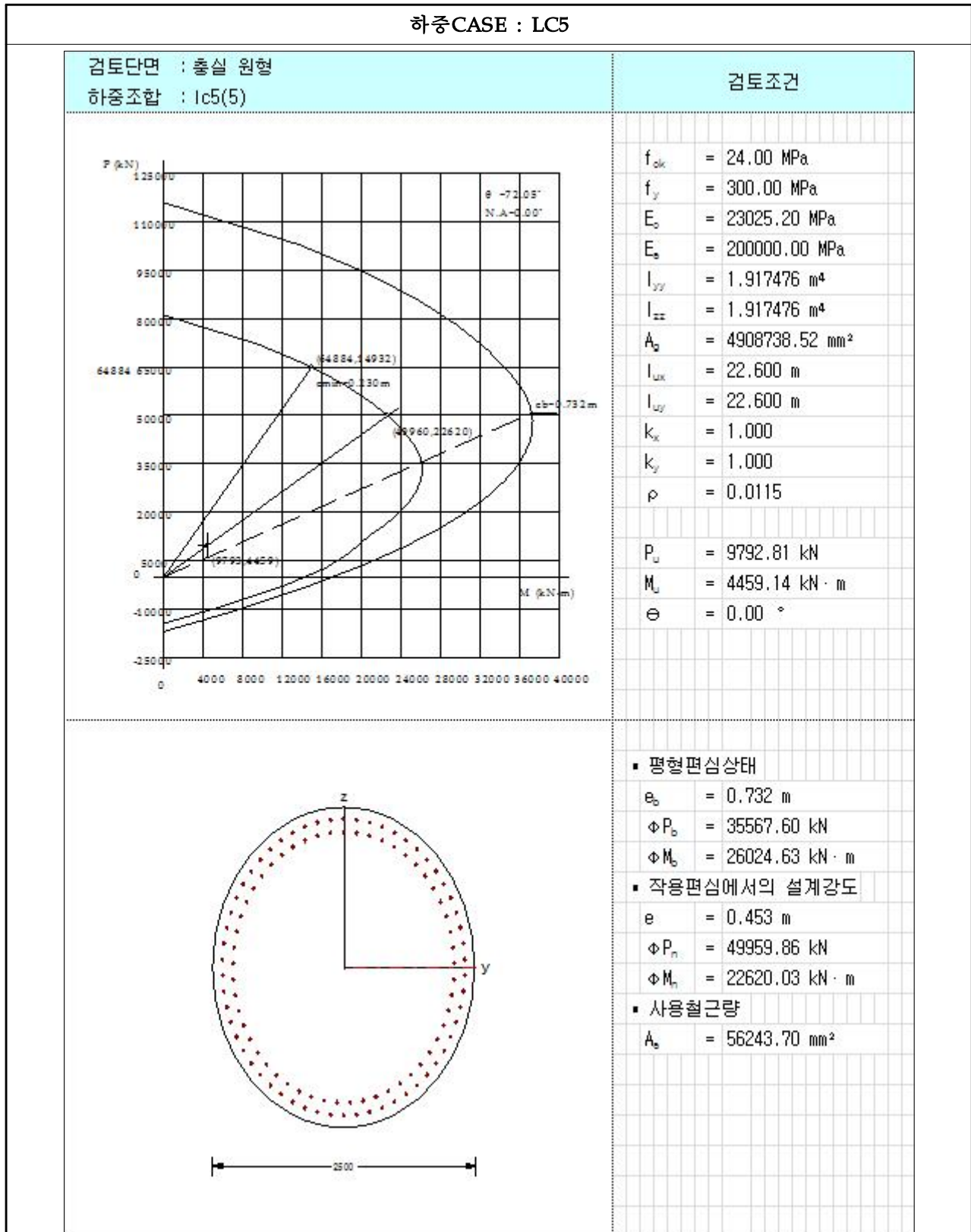
【그림 6.4.36】 P-M 상관도(하중CASE : LC5)(부산)
