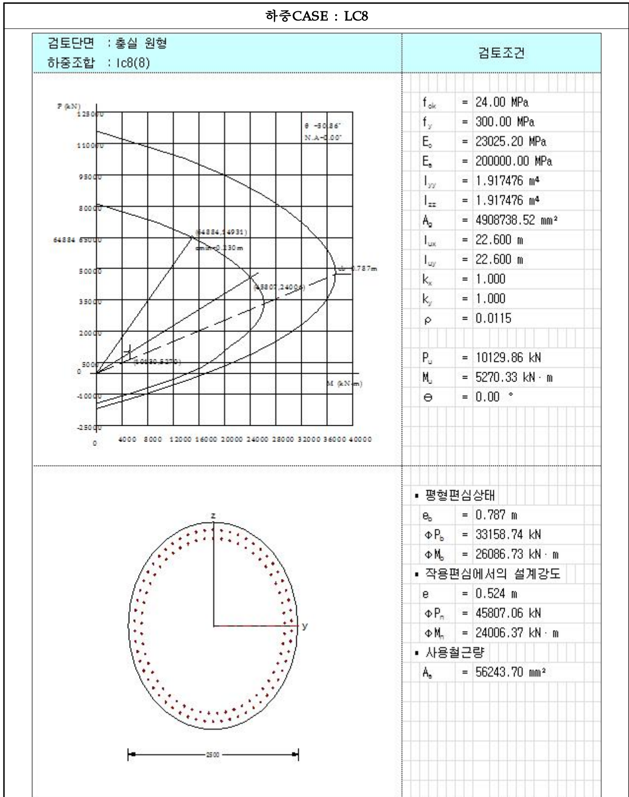
【그림 6.4.30】 P-M 상관도(하중CASE : LC8)(부산)
