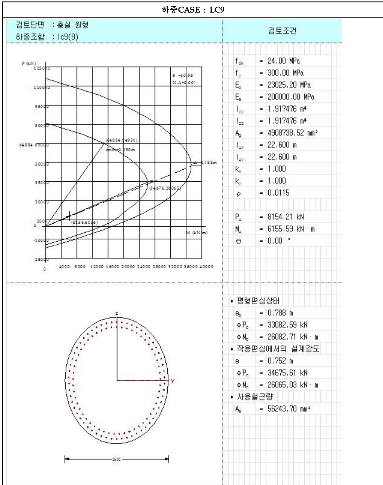
【그림 6.440】 P-M 상관도(하중CASE : LC9)(부산)
