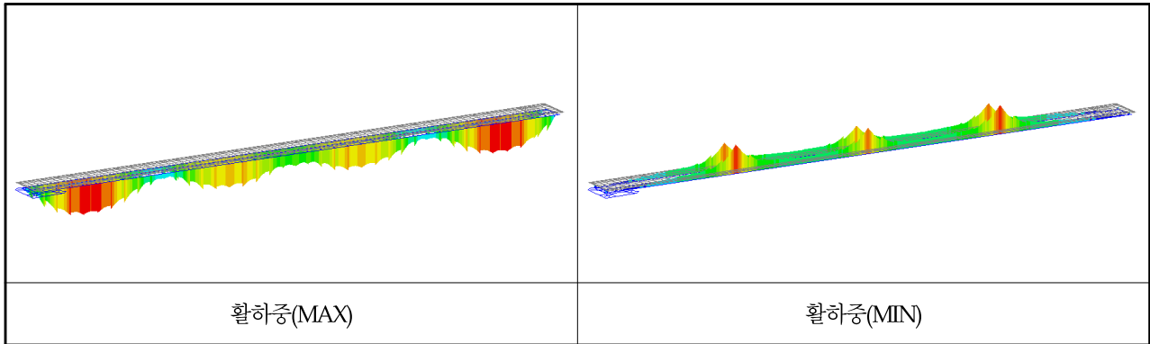
【그림 6.2.7】 휨모멘트도(대구,계속)
