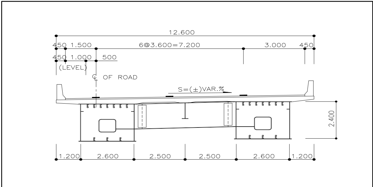
【그림 6.2.13】 해석단면(부산)
