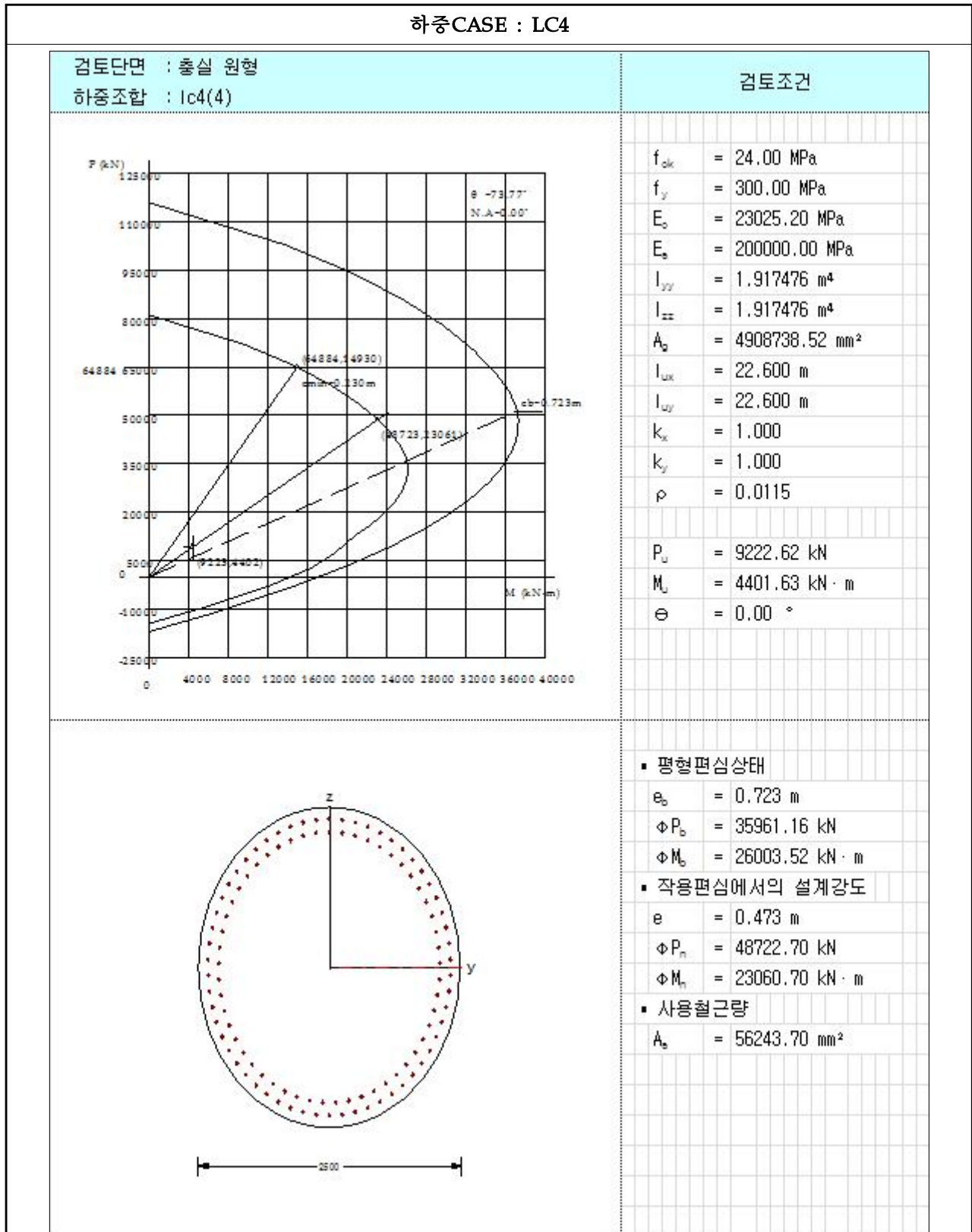
【그림 6.4.6】 P-M 상관도(하중CASE : LC4)(대구)
