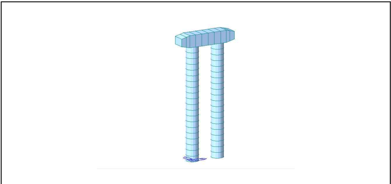
【그림 6.4.2】 해석모델링(P6)(대구)
