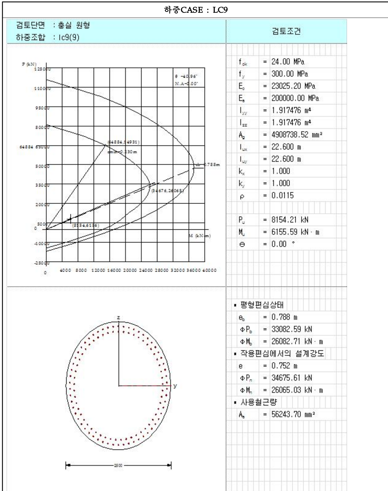
【그림 6.4.20】 P-M 상관도(하중CASE : LC9)(대구)
