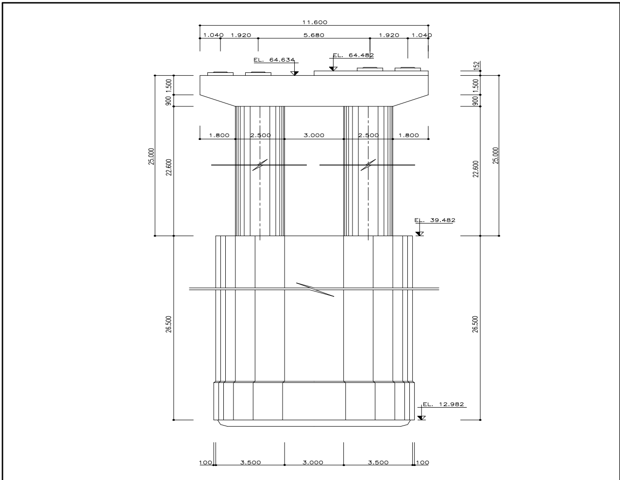
【그림 6.4.21】 해석단면(P6)(부산)
