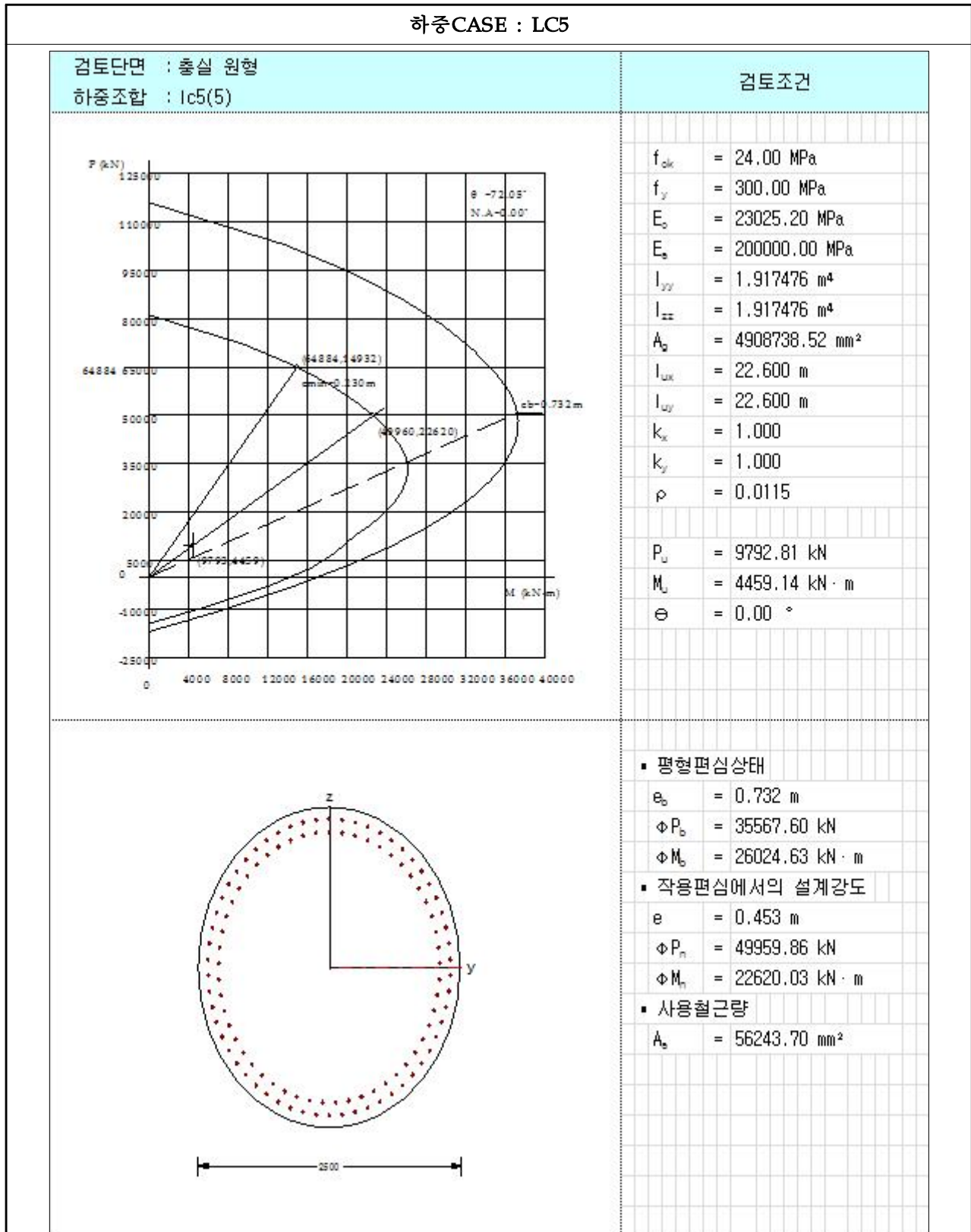
【그림 6.4.27】 P-M 상관도(하중CASE : LC5)(부산)
