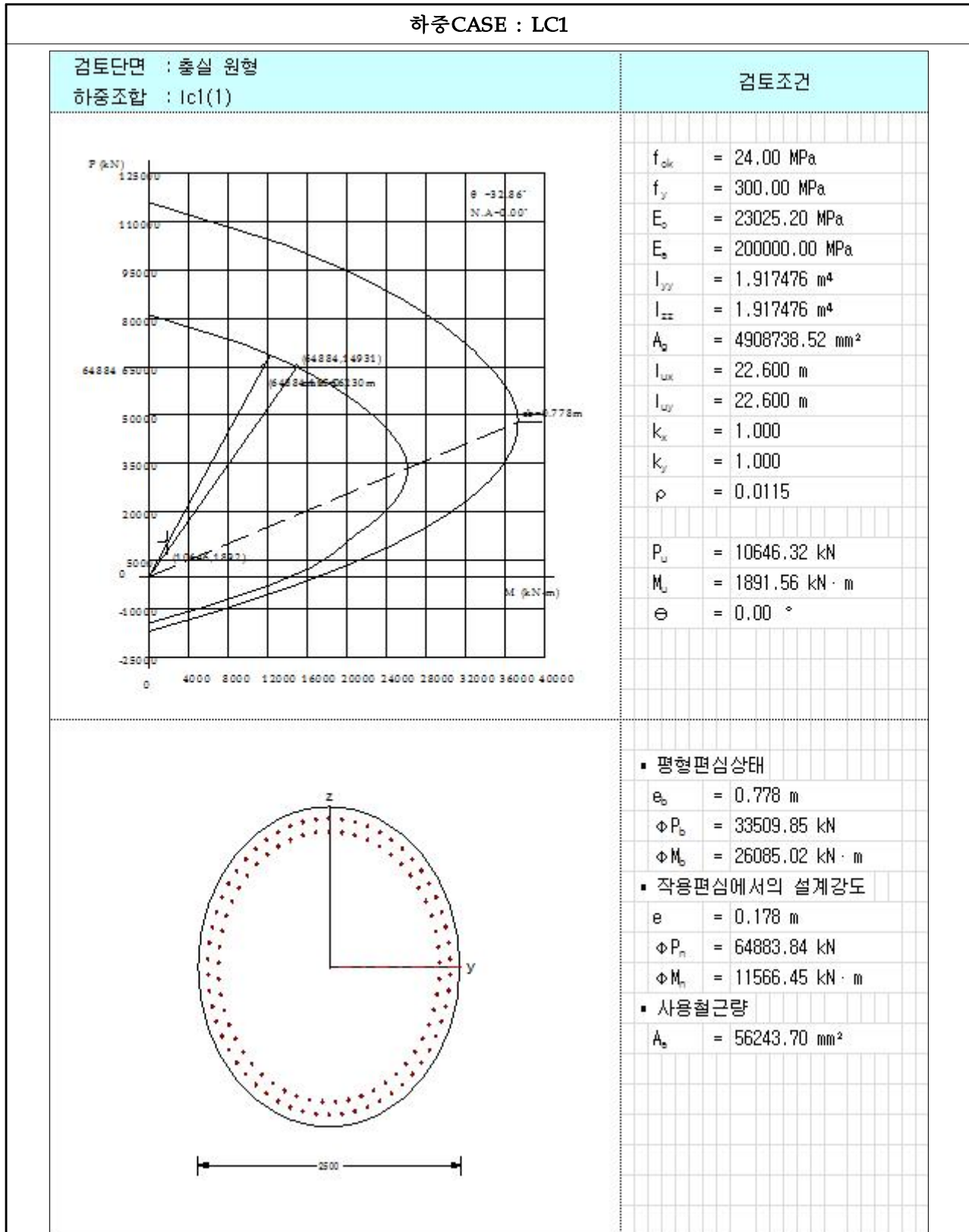
【그림 6.4.3】 P-M 상관도(하중CASE : LC1)(대구)
