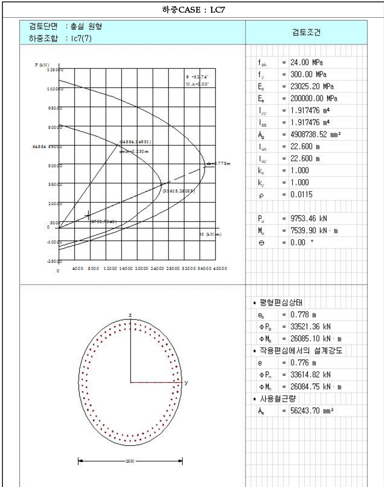
【그림 6.4.9】 P-M 상관도(하중CASE : LC7)(대구)
