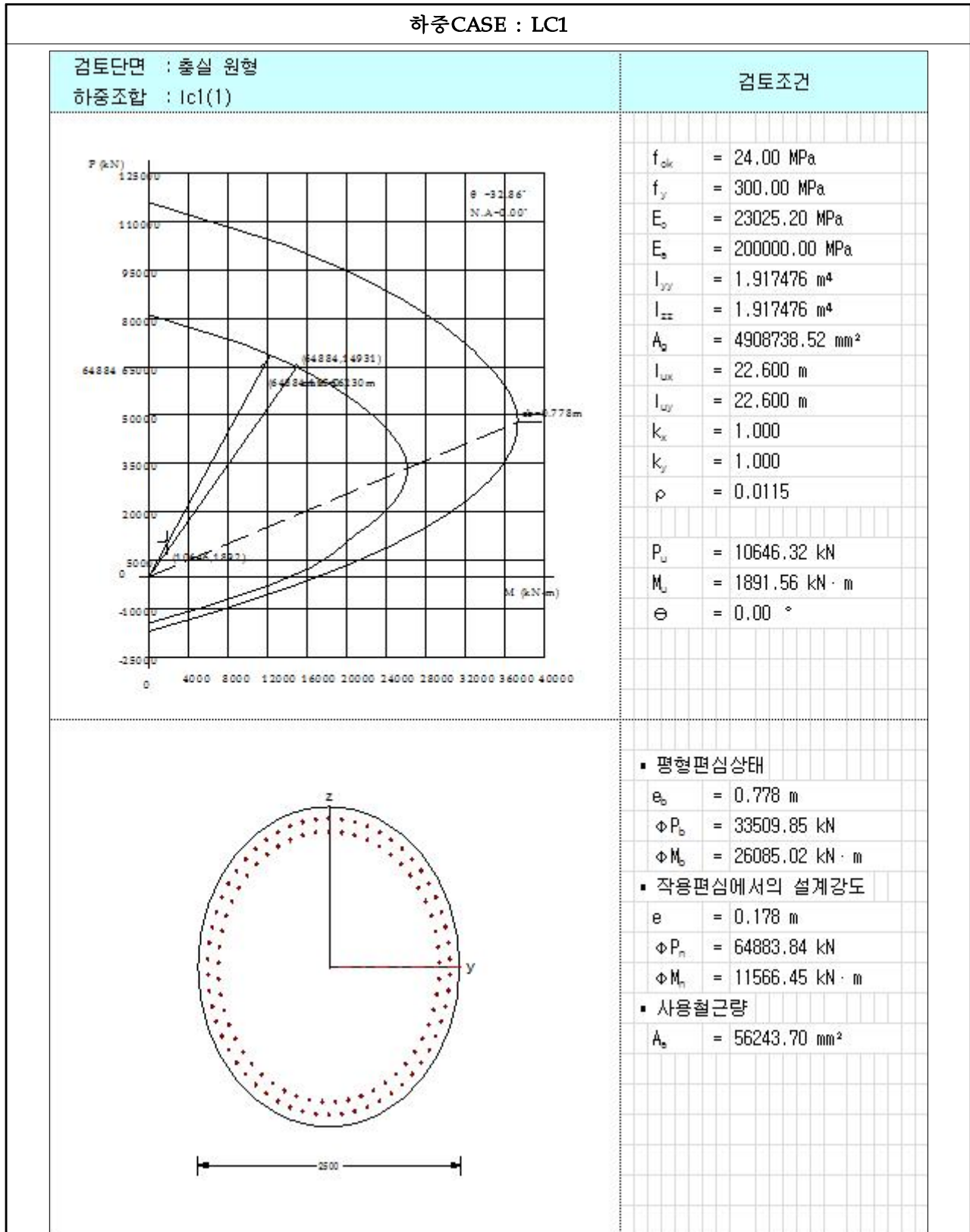
【그림 6.4.23】 P-M 상관도(하중CASE : LC1)(부산)
