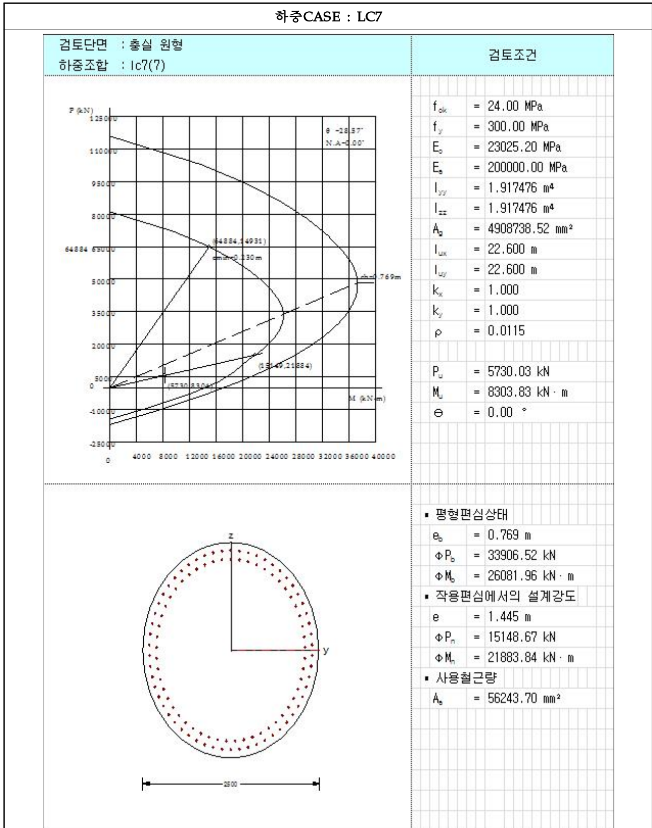
【그림 6.4.18】 P-M 상관도(하중CASE : LC7)(대구)
