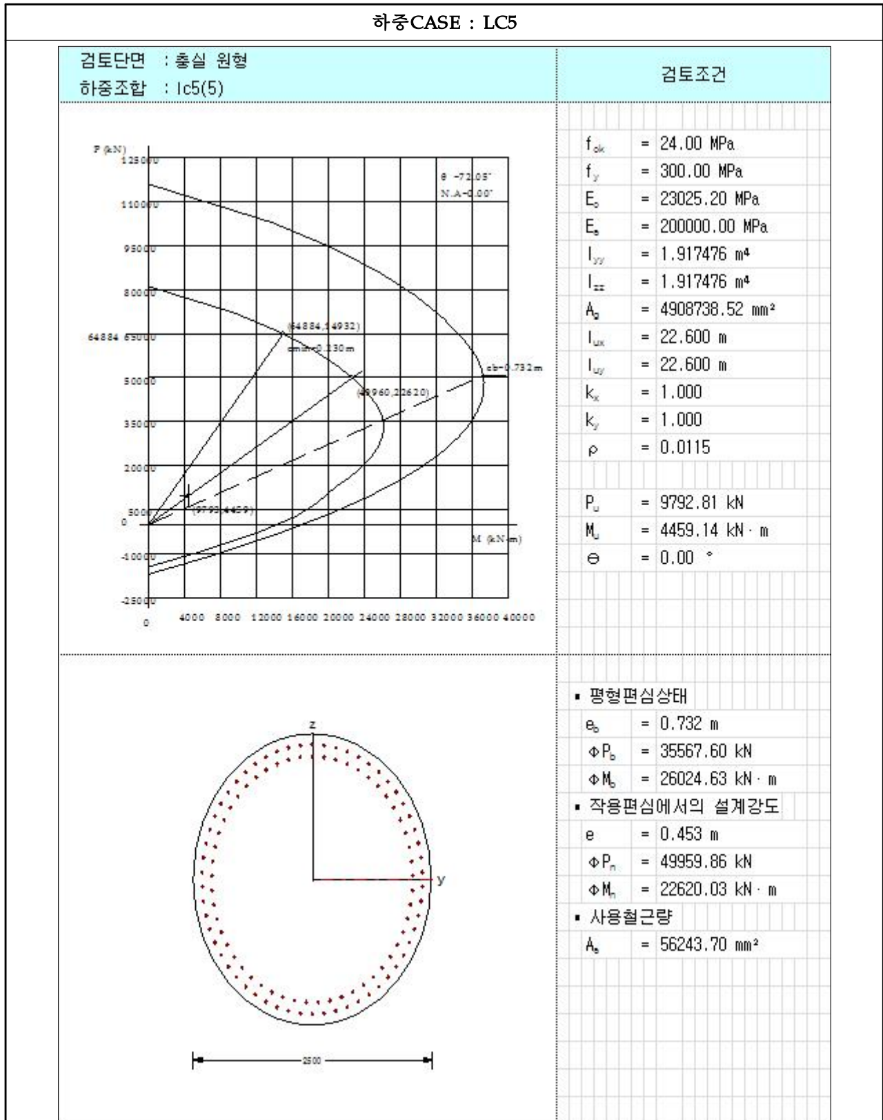
【그림 6.4.16】 P-M 상관도(하중CASE : LC5)(대구)
