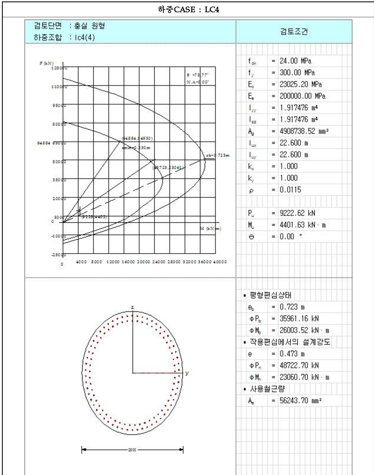
【그림 6.4.15】 P-M 상관도(하중CASE : LC4)(대구)
