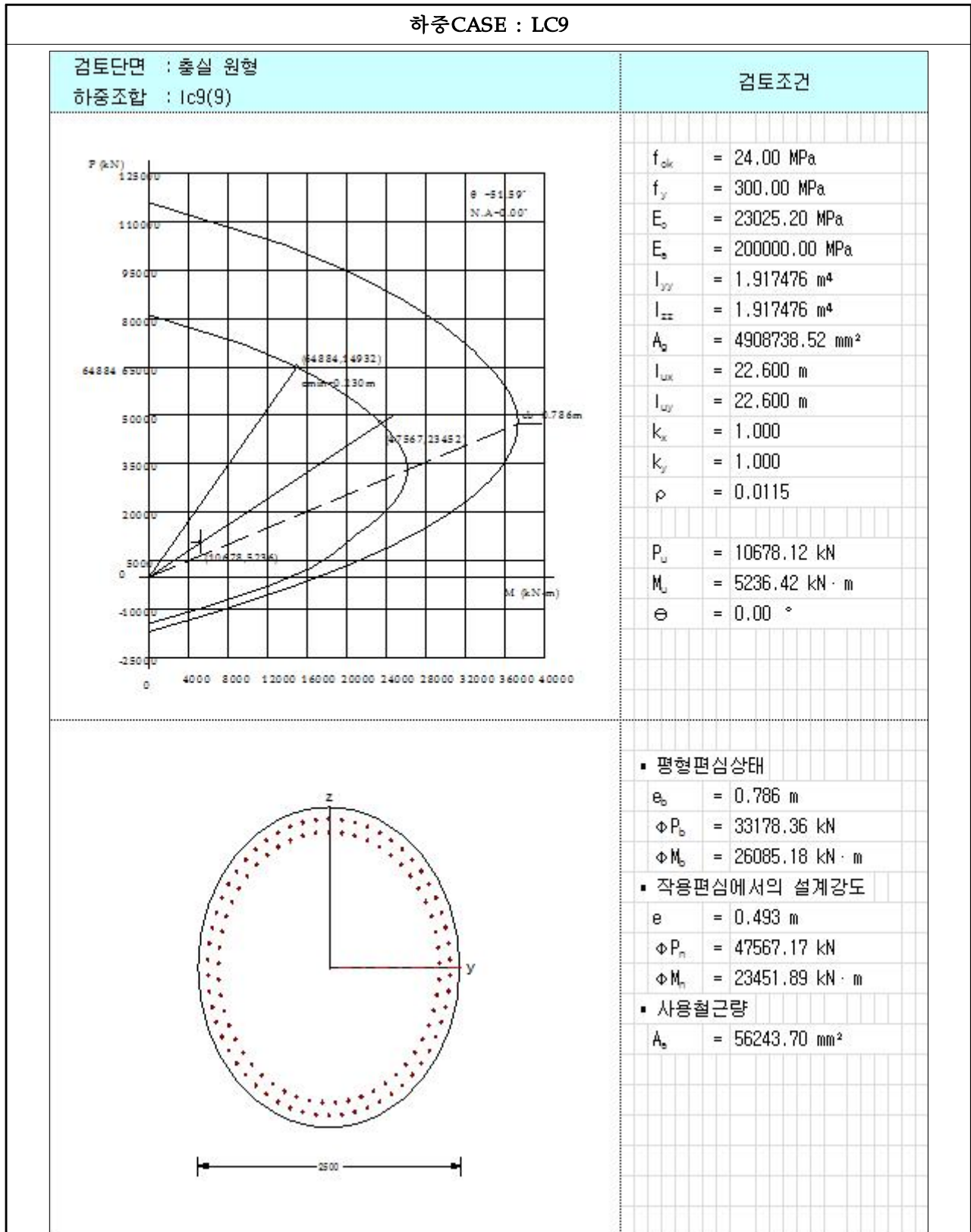
【그림 6.4.31】 P-M 상관도(하중CASE : LC9)(부산)
