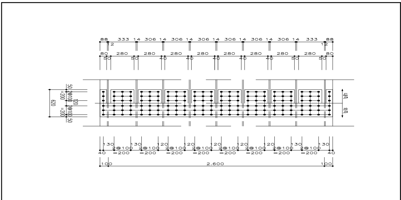
【그림 6.2.9】 압축부 플랜지 이음(대구)
