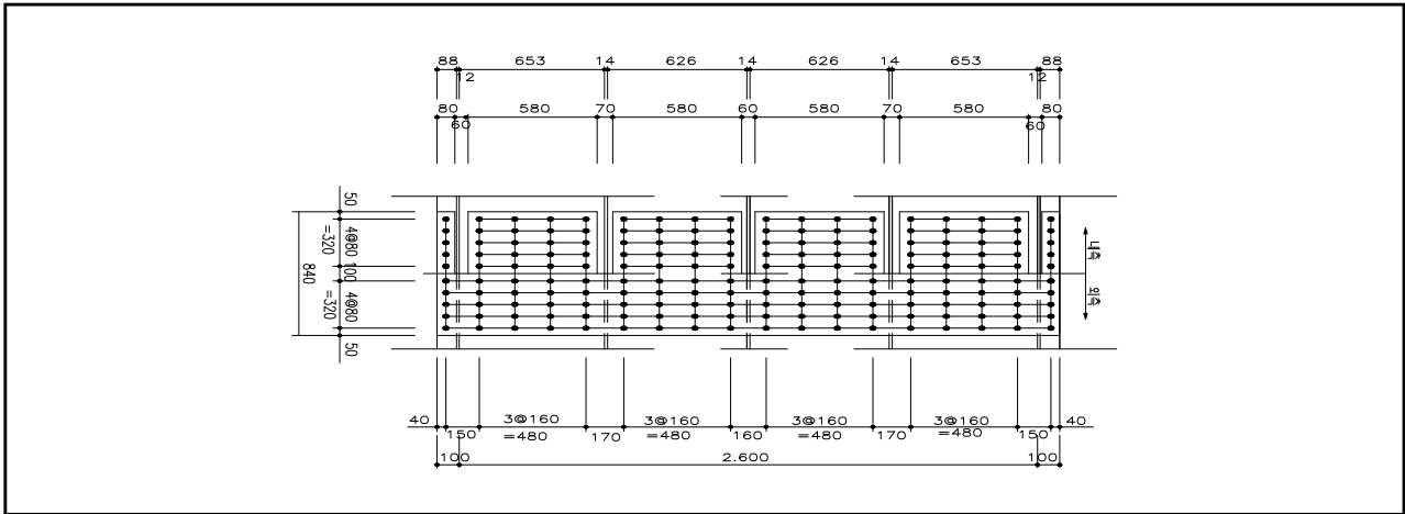
【그림 6.2.22】 인장부 플랜지 이음(부산)
