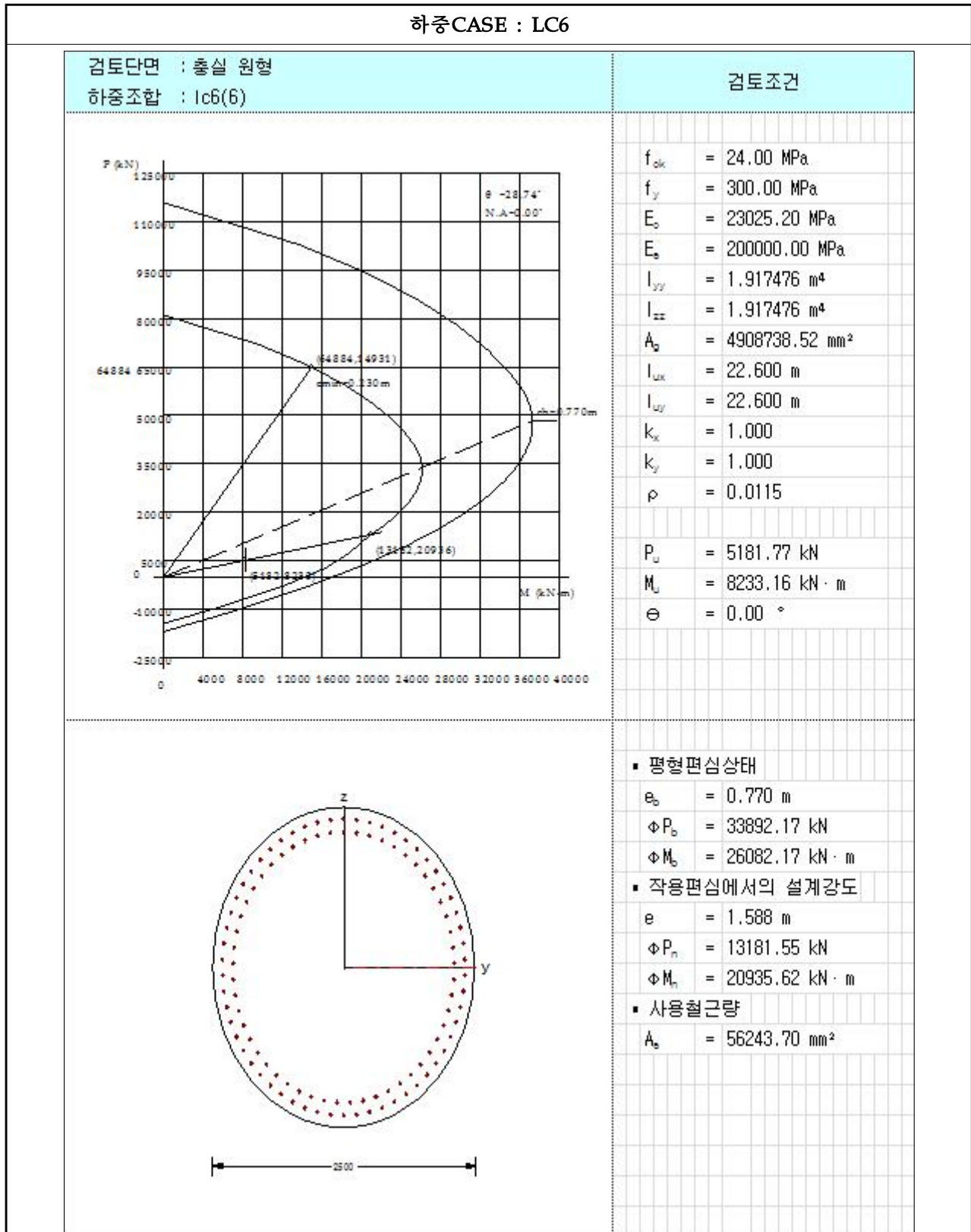
【그림 6.4.37】 P-M 상관도(하중CASE : LC6)(부산)
