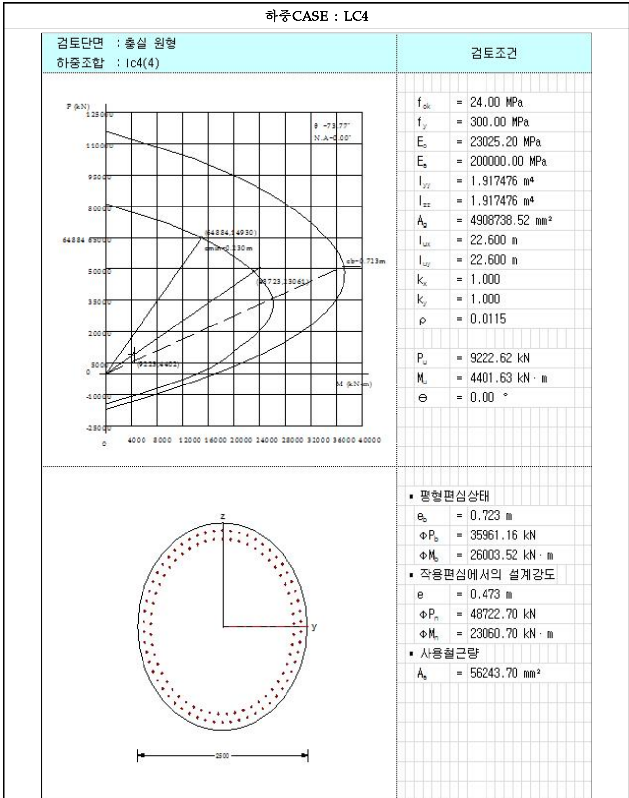
【그림 6.4.35】 P-M 상관도(하중CASE : LC4)(부산)
