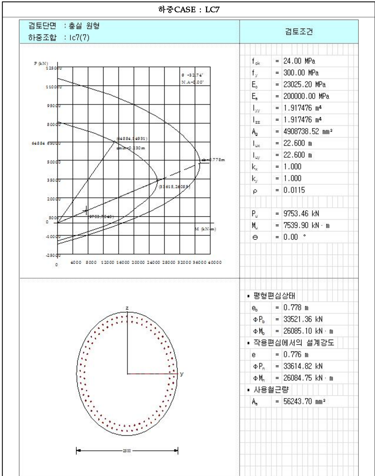
【그림 6.4.29】 P-M 상관도(하중CASE : LC7)(부산)
