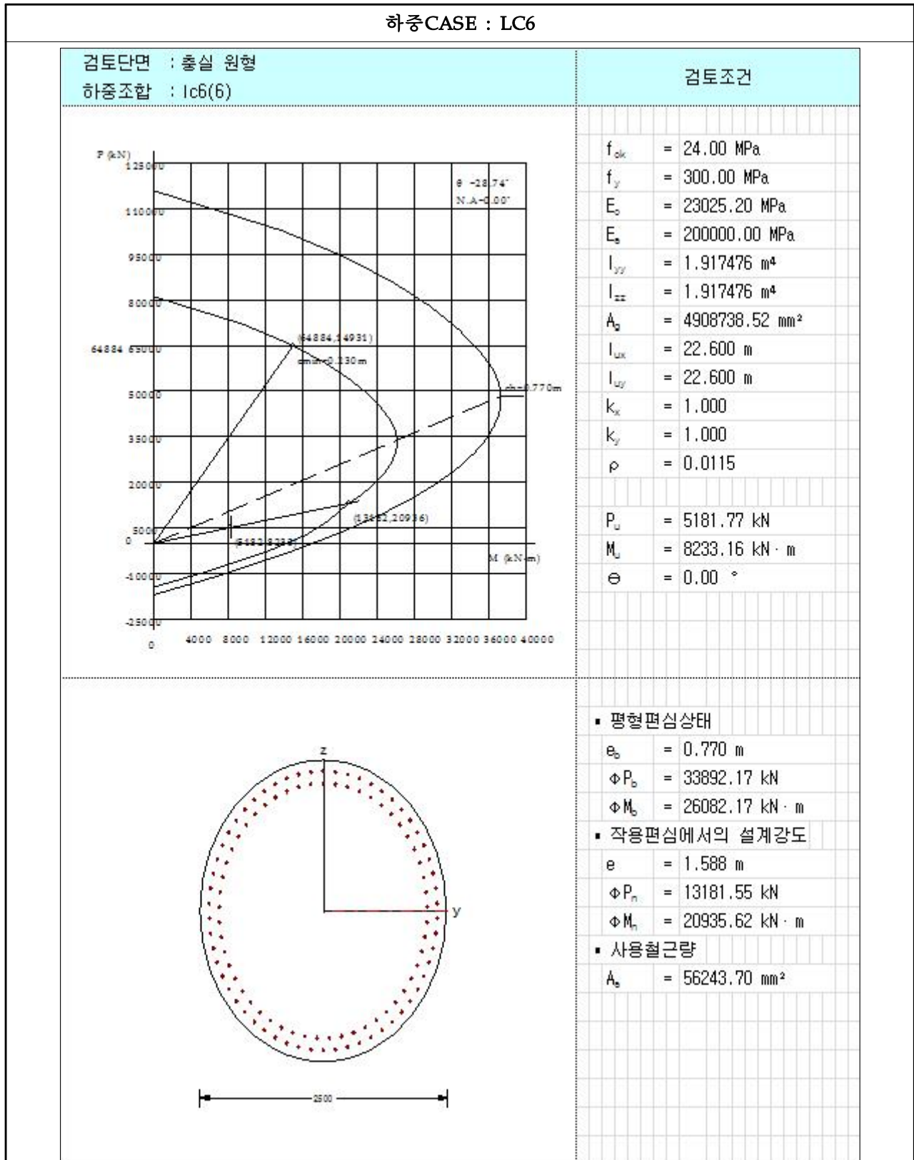
【그림 6.4.17】 P-M 상관도(하중CASE : LC6)(대구)
