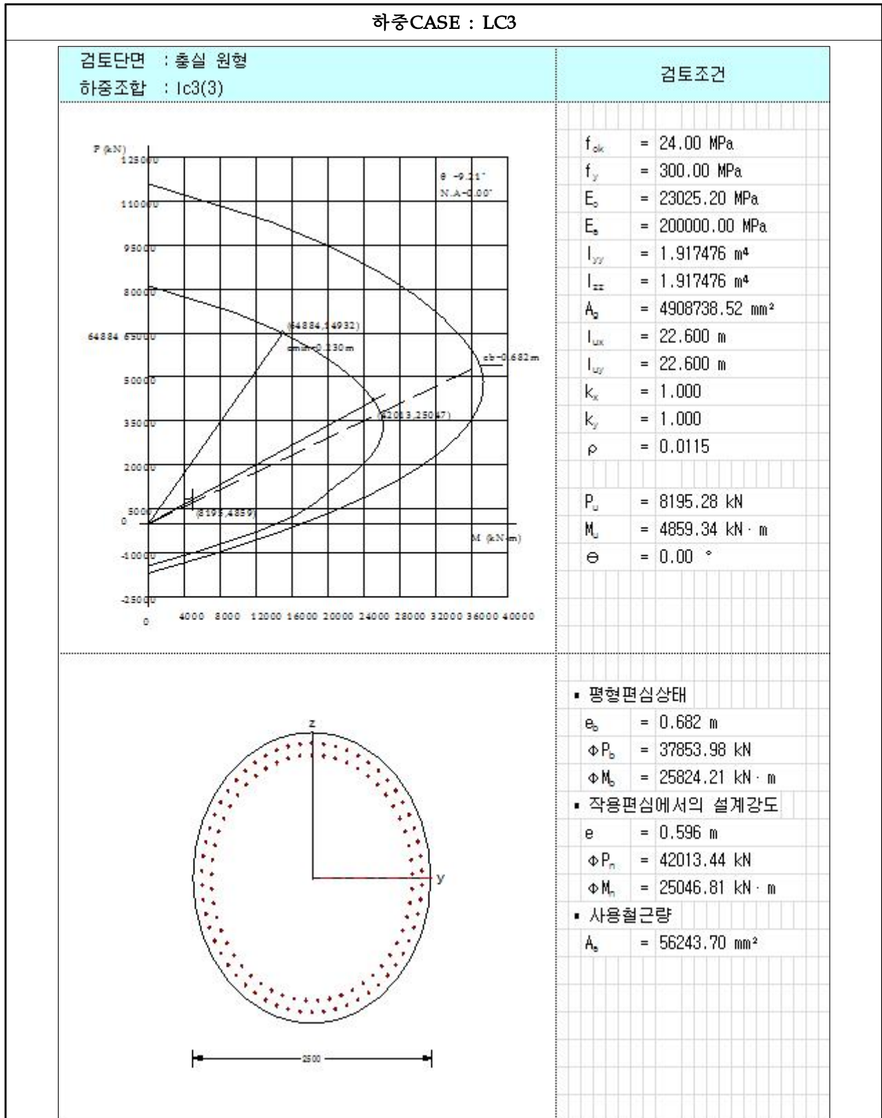
【그림 6.4.34】 P-M 상관도(하중CASE : LC3)(부산)
