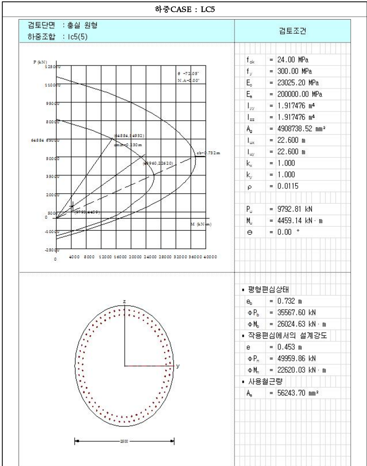
【그림 6.4.7】 P-M 상관도(하중CASE : LC5)(대구)
