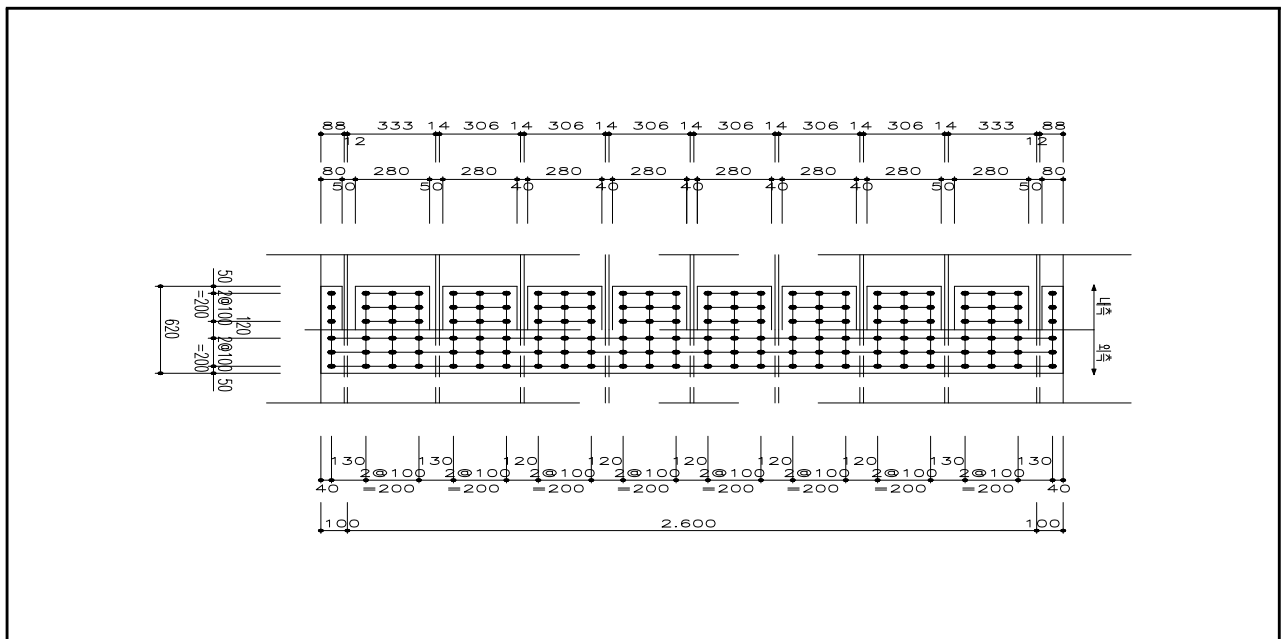
【그림 6.2.21】 압축부 플랜지 이음(부산)
