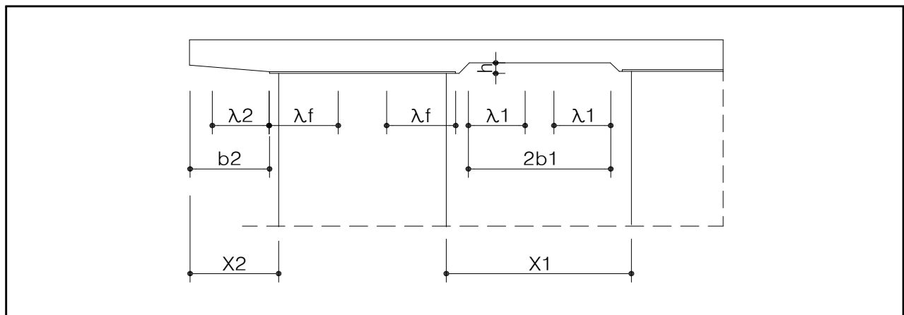
【그림 6.2.16】 바닥판의 유효폭(부산)
