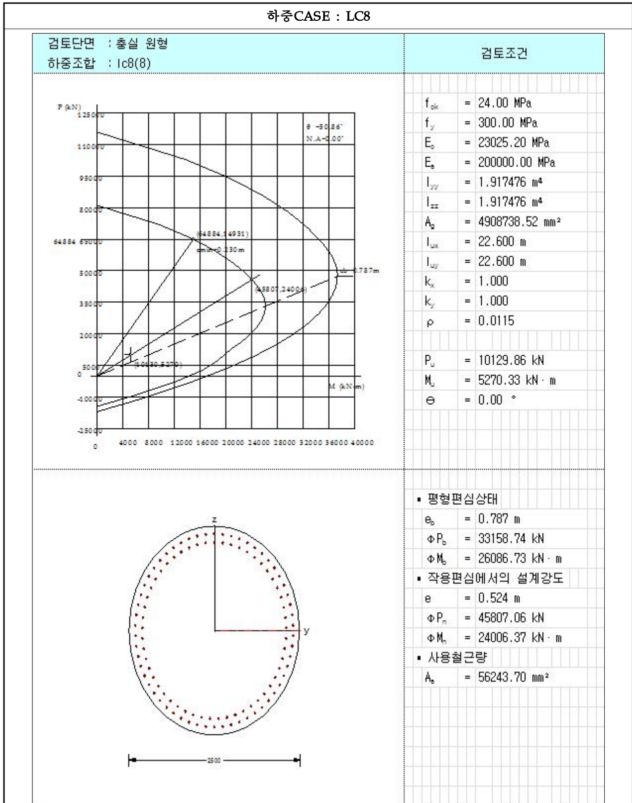
【그림 6.4.10】 P-M 상관도(하중CASE : LC8)(대구)
