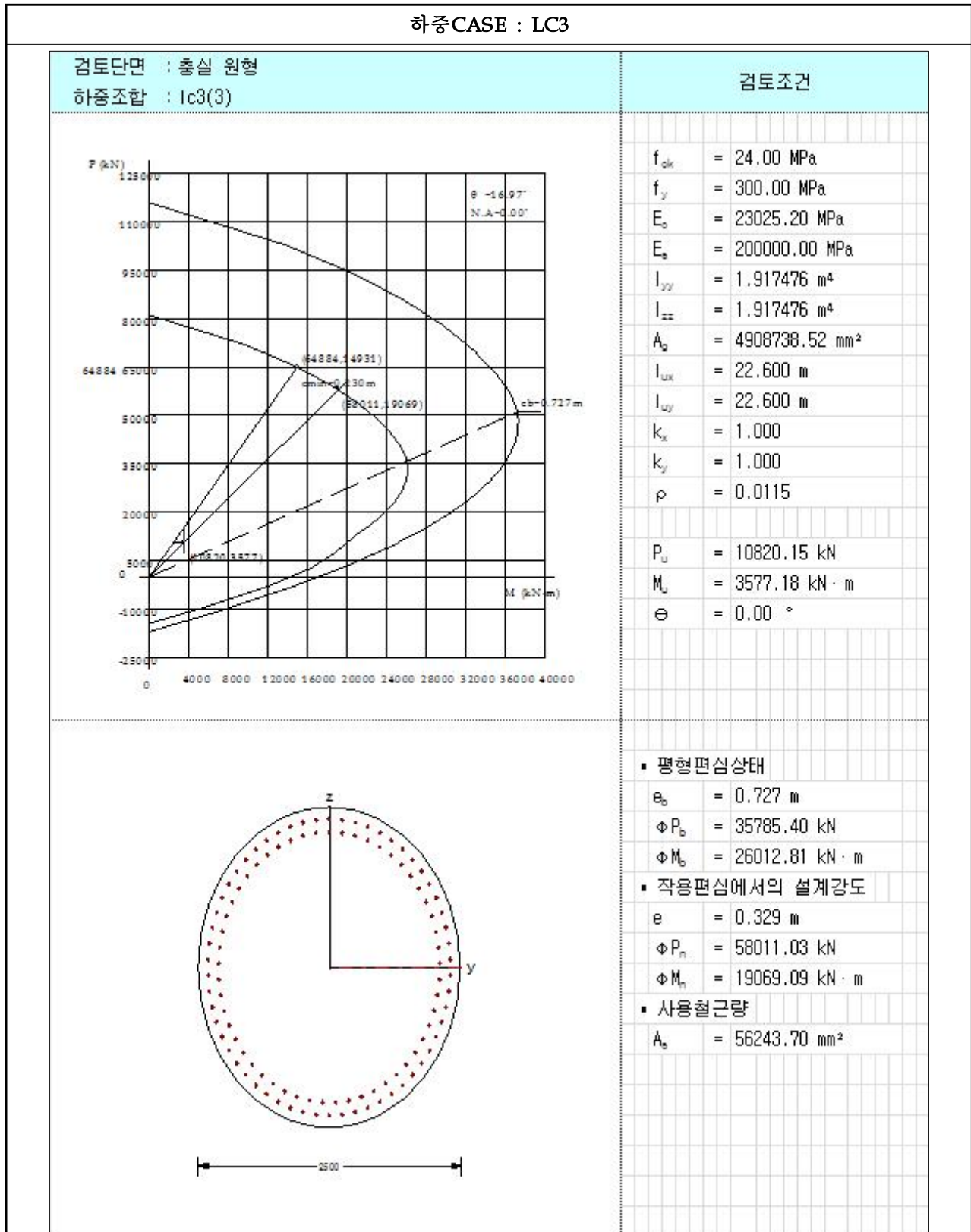
【그림 6.4.25】 P-M 상관도(하중CASE : LC3)(부산)
