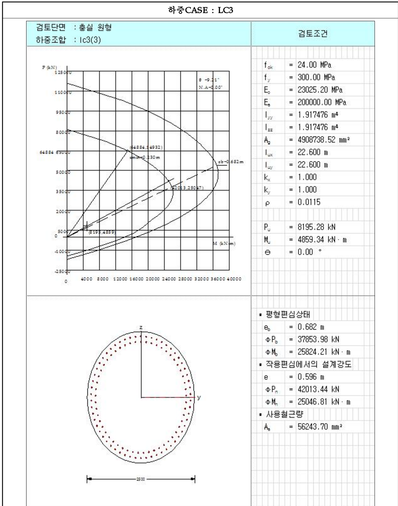
【그림 6.4.14】 P-M 상관도(하중CASE : LC3)(대구)
