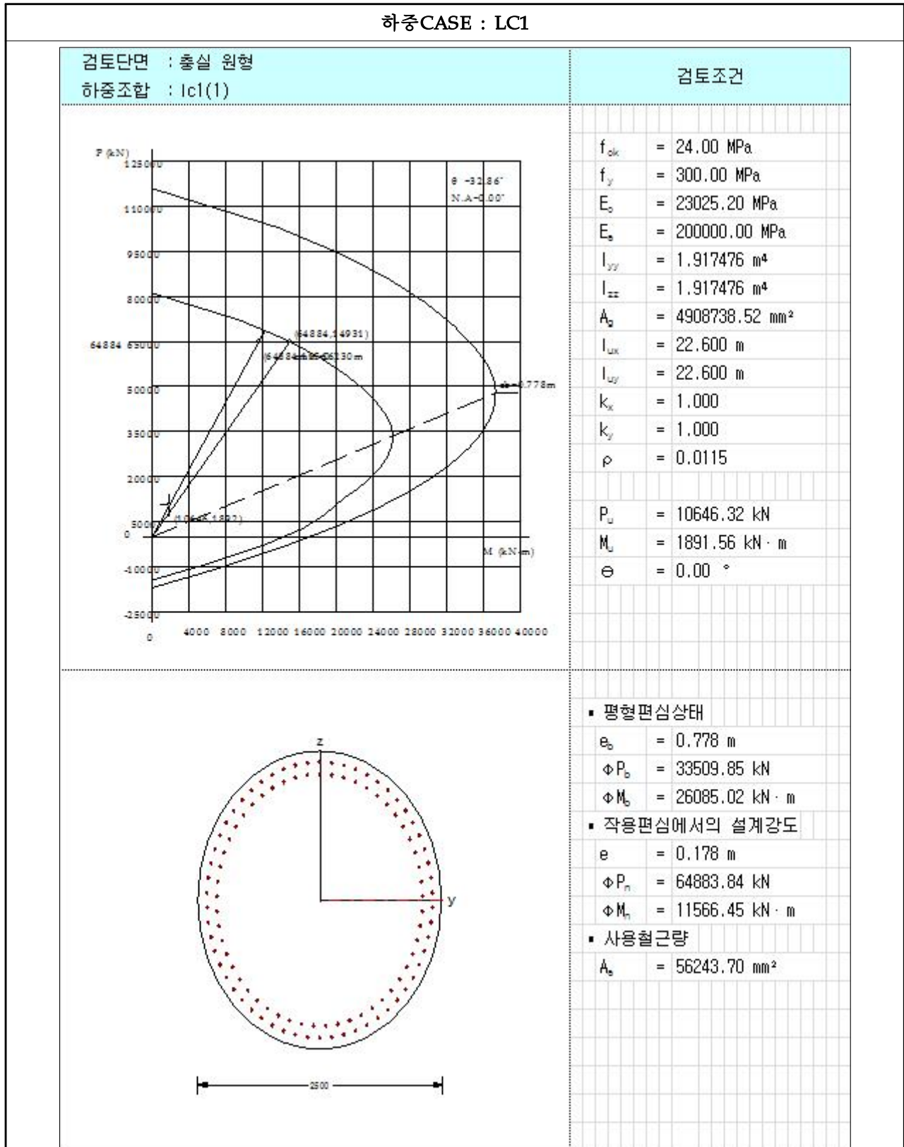
【그림 6.432】 P-M 상관도(하중CASE : LC1)(부산)
