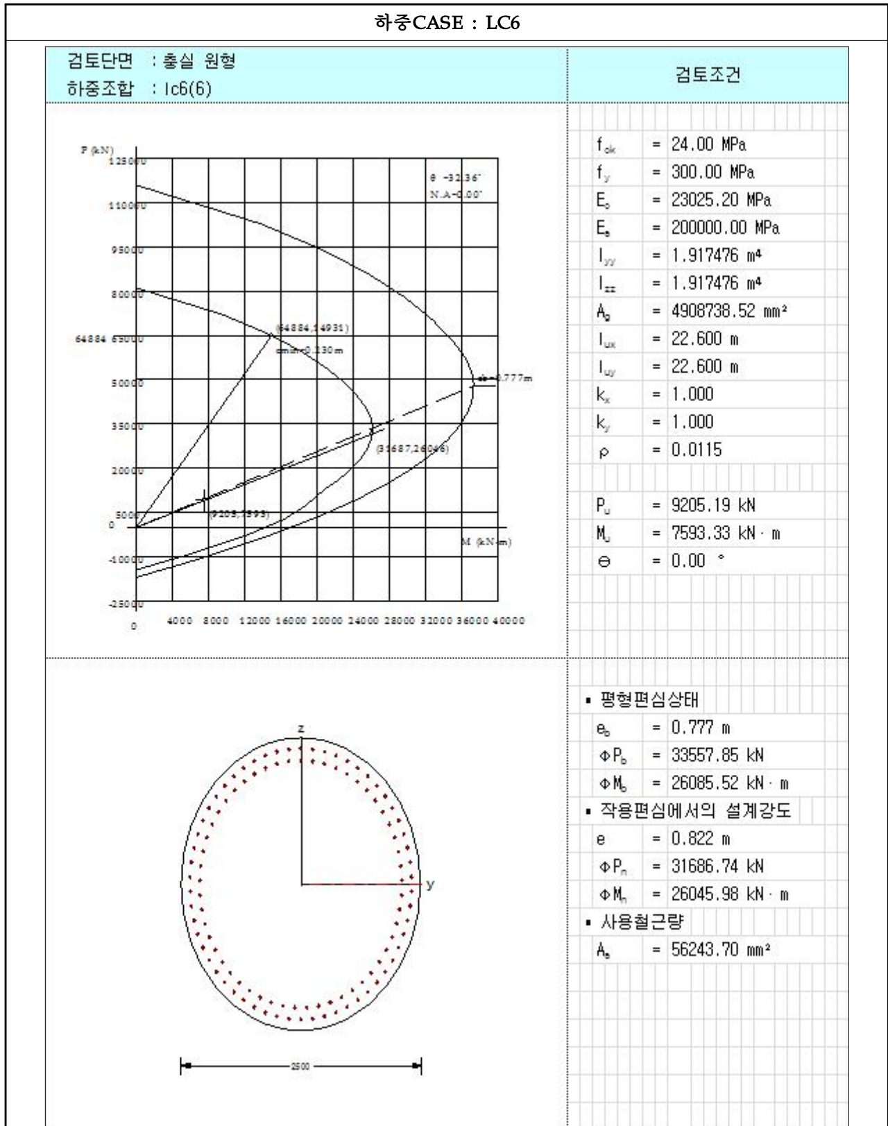
【그림 6.4.28】 P-M 상관도(하중CASE : LC6)(부산)
